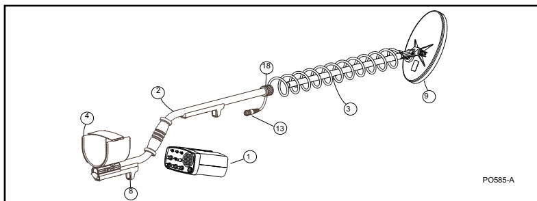
Figura 4 - Montaje completo de la barra
