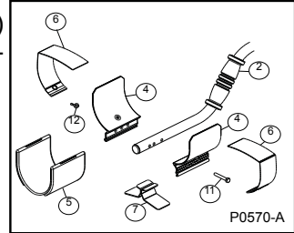
Figura 2 - Apoyabrazos/ barra superior
